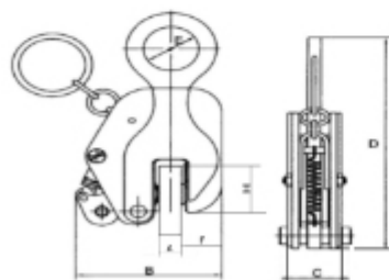
Рисунок 3. Размеры захвата
